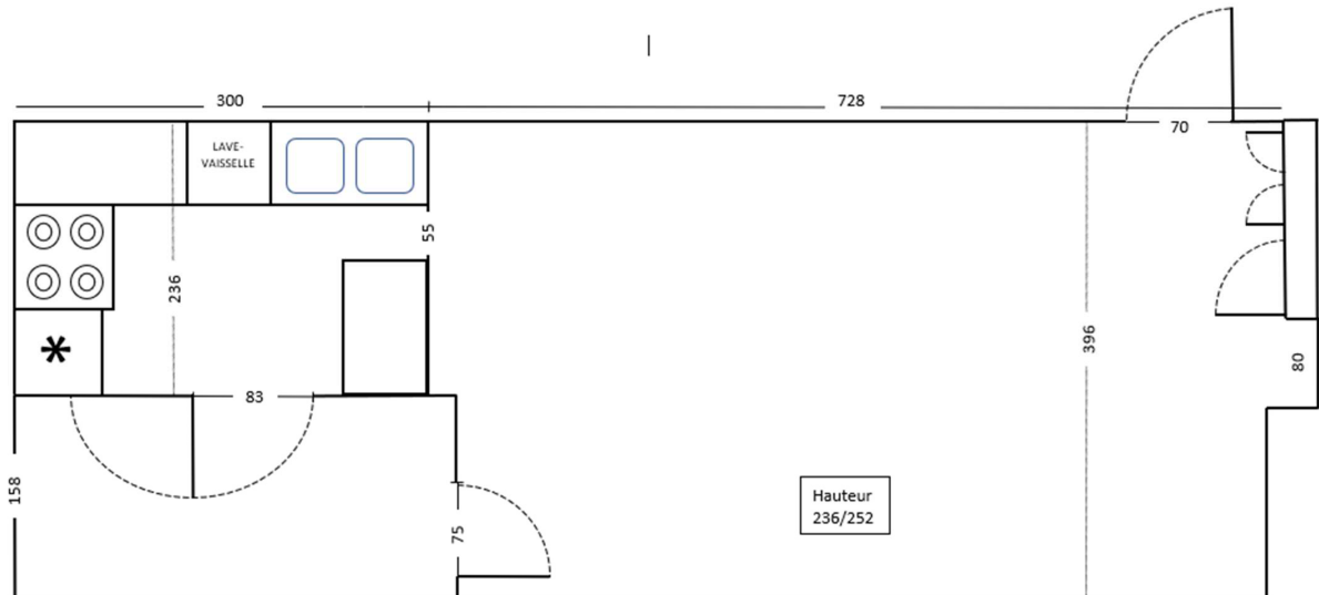
PLAN DE LA CANTINE MOBILE
